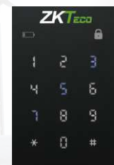
Random Digit
